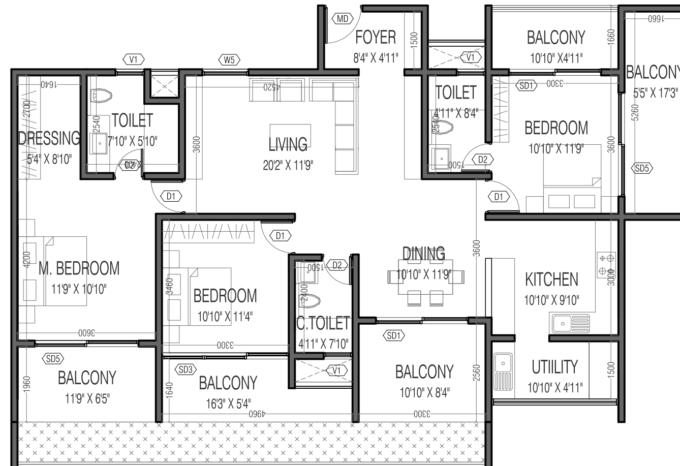
3BHK TYPE 1C
