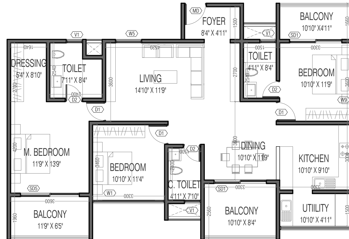
3BHK TYPE 1A
